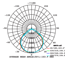
Ljuskurva 10-7002
