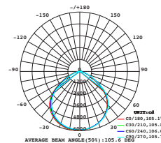
Ljuskurva 10-7003
