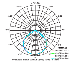
Ljuskurva 10-7004
