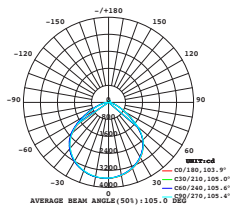
Ljuskurva 10-7001
